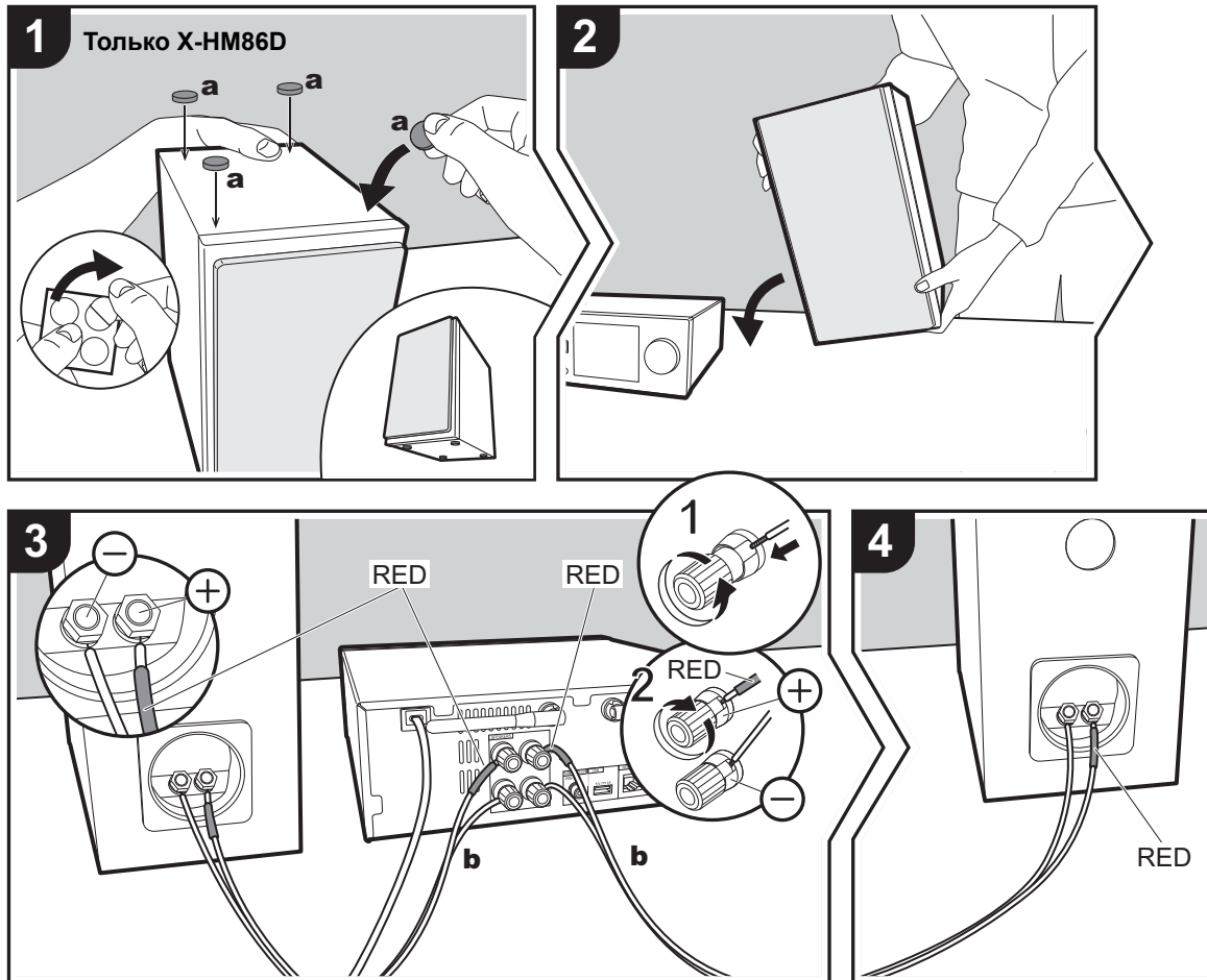
a Противоскользящие подкладки, b Кабели для AC
